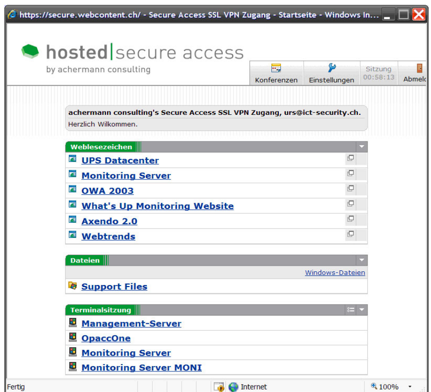
Beispiel: individuelle Benutzerkonsole im Browserfenster
